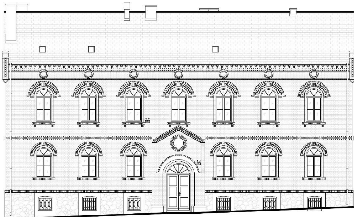
ELEWACJA FRONTOWA
