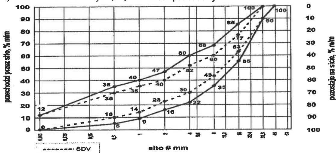
Rysunek 3. Mieszanka kruszyw 0/31,5 do warstw podbudowy
